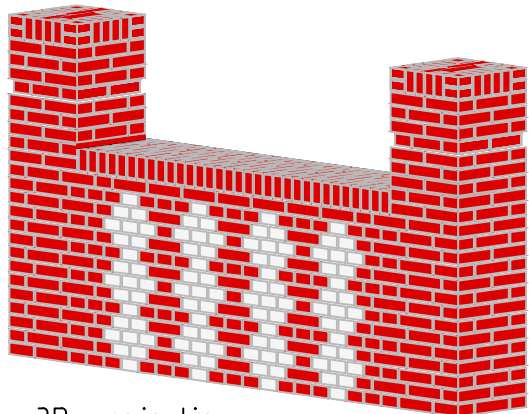
3D projectie
