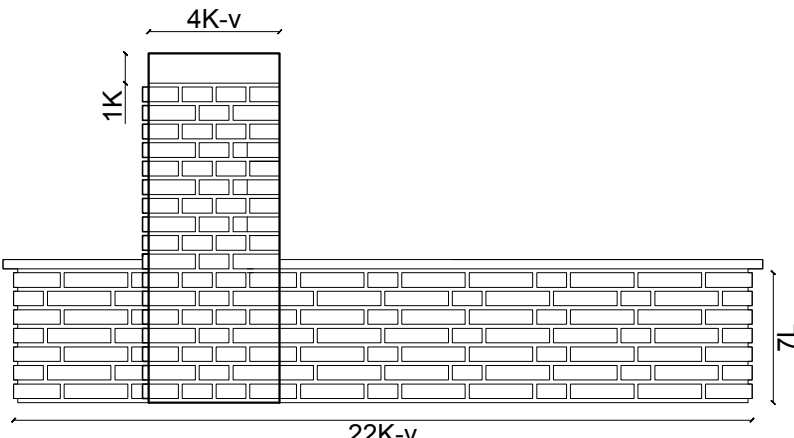
Achteraanzicht
