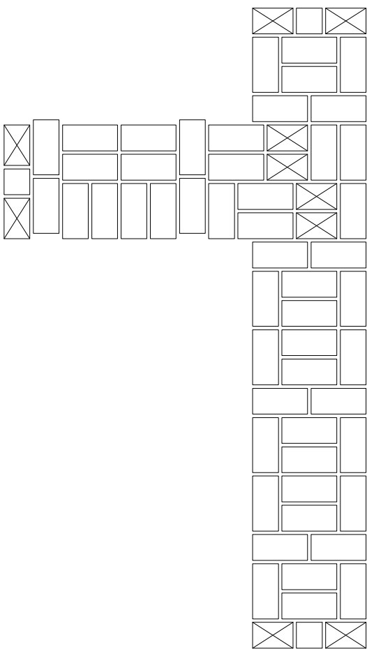
Lagen 2, 4, 6
