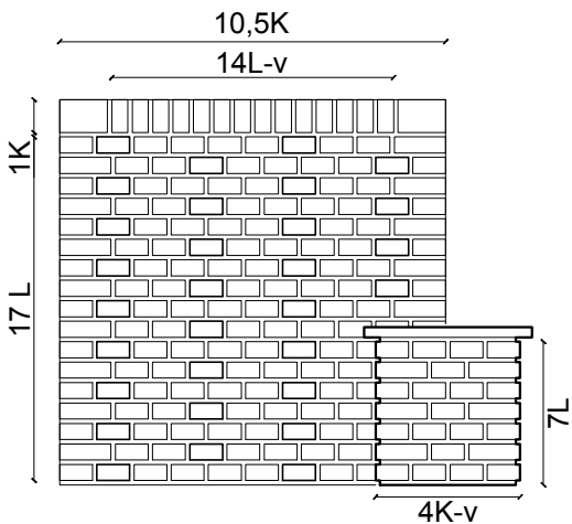
Zijaanzicht Zuid
