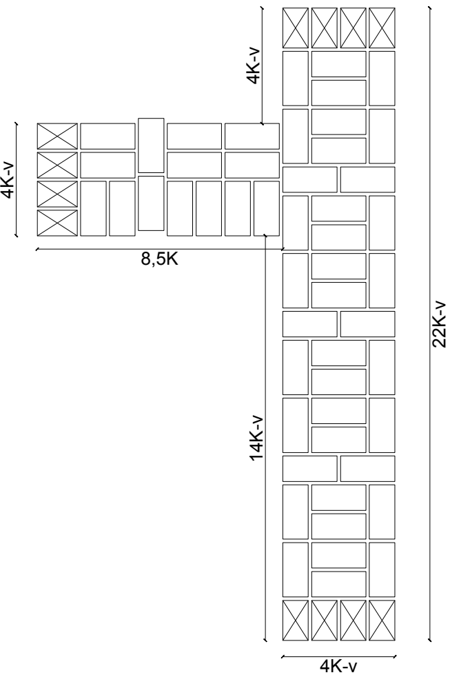
Lagen 1, 3, 5, 7
