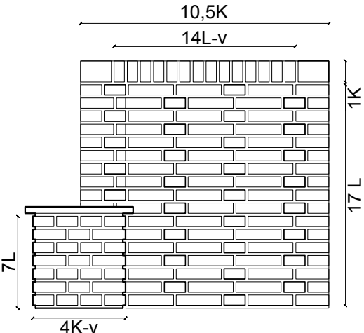
Zijaanzicht Noord
