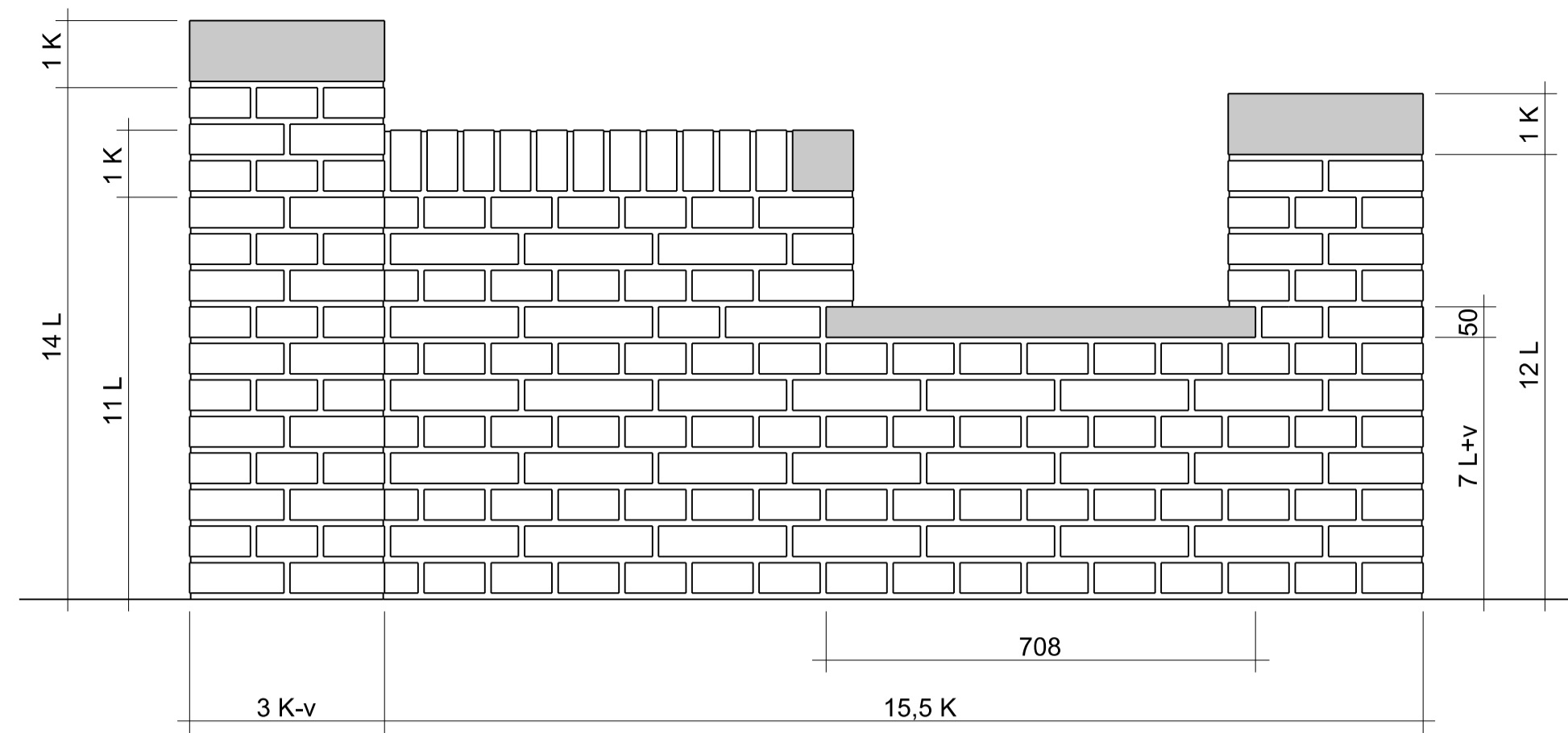
VOORAANZICHT
