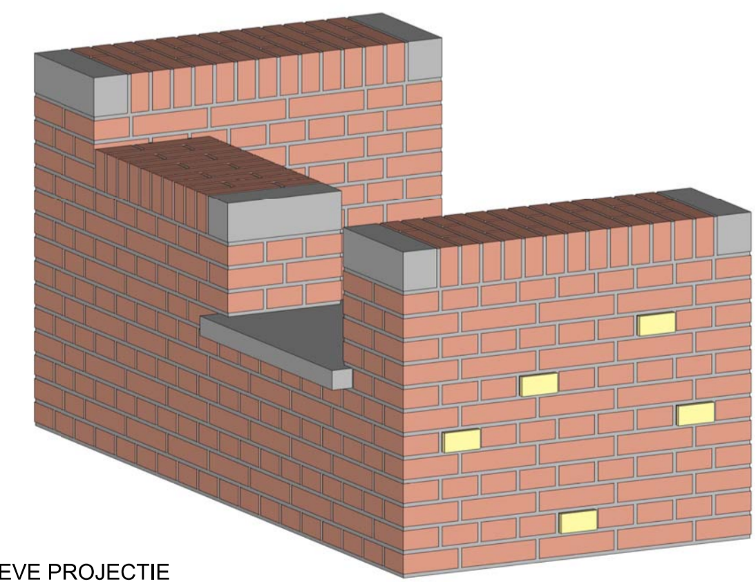
SCHEVE PROJECTIE
