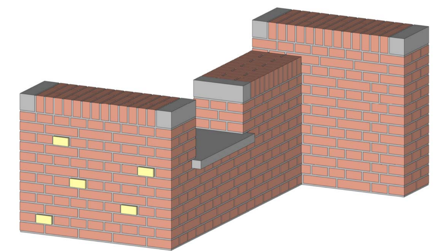
SCHEVE PROJECTIE
