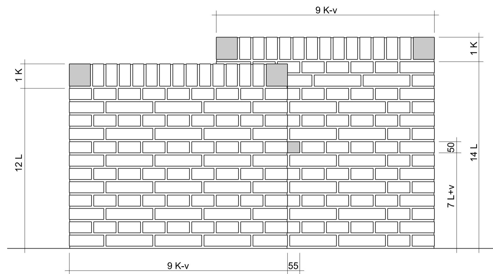
ZIJUAANZICHT
