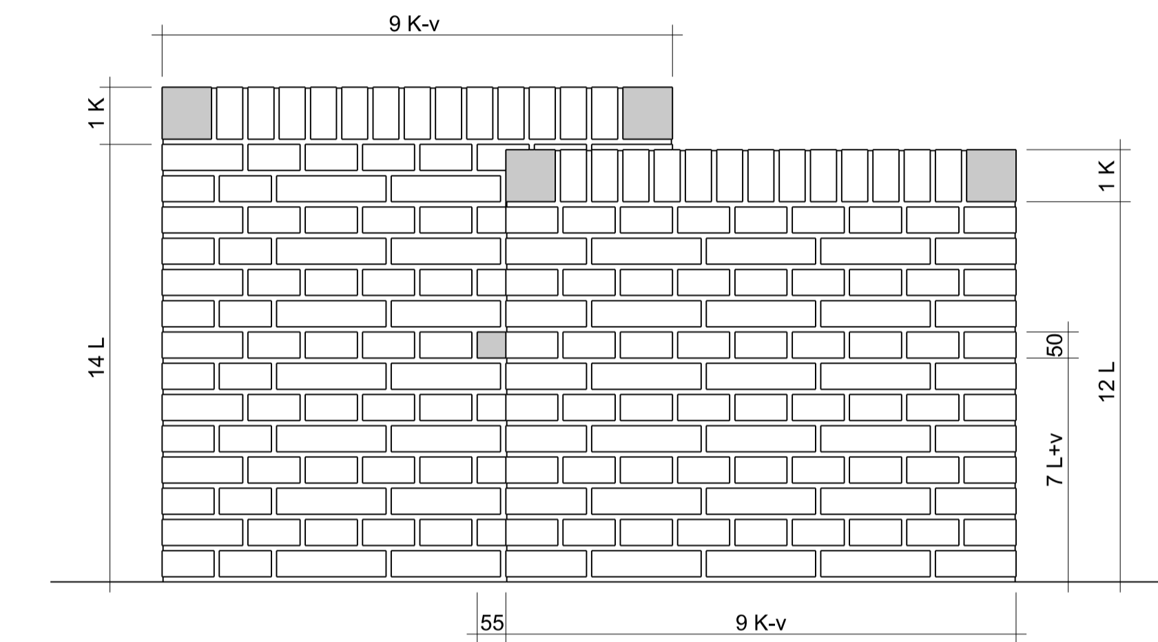
ZIJAAANZICHT
