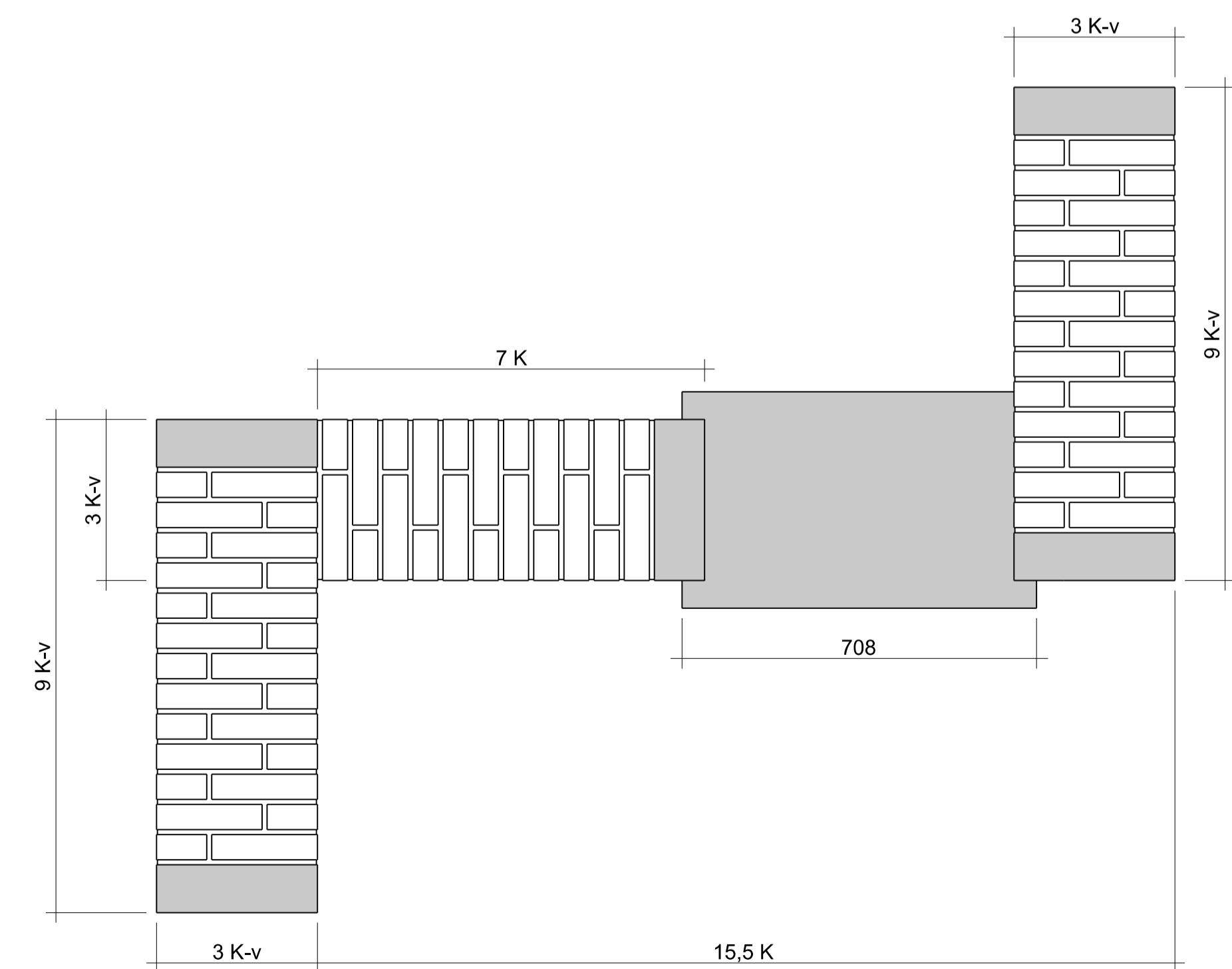
BOVENAANZICHT
