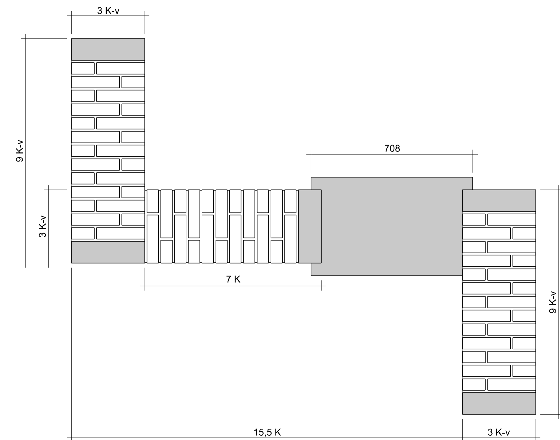
BOVENAANZICHT
