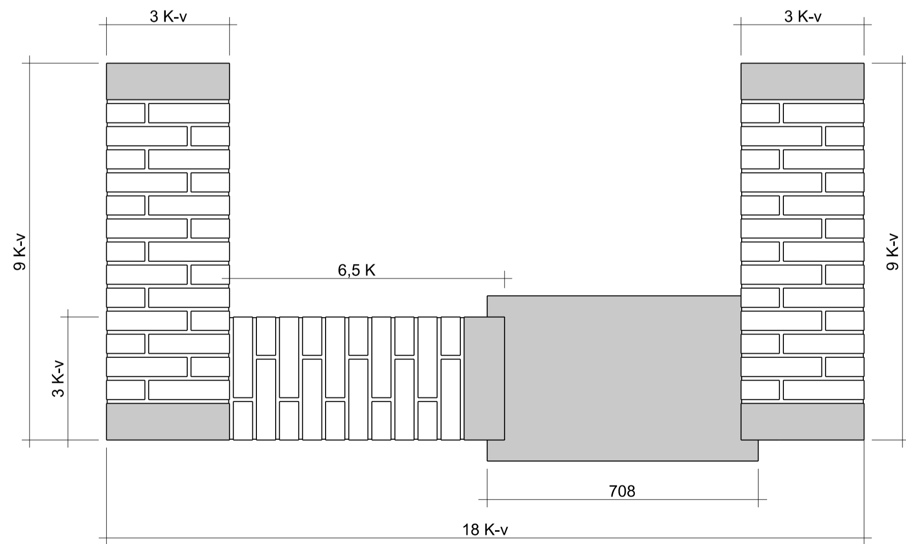
BOVENAANZICHT
