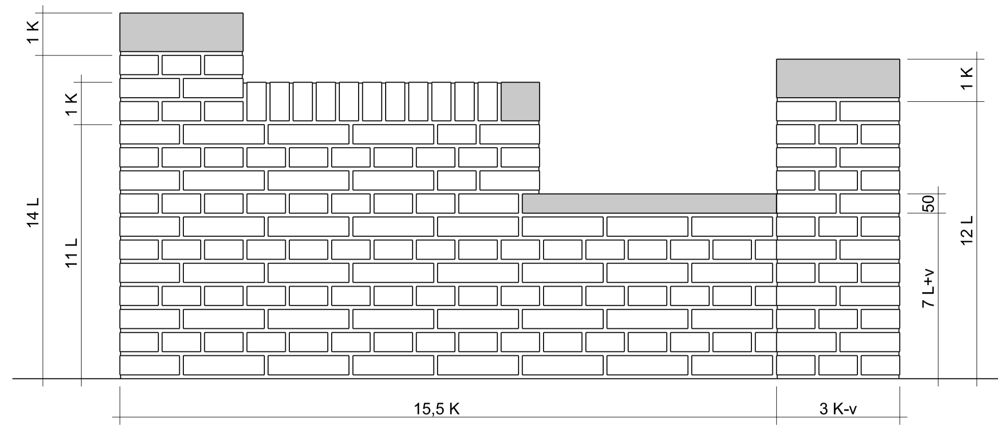
VOORAANZICHT
