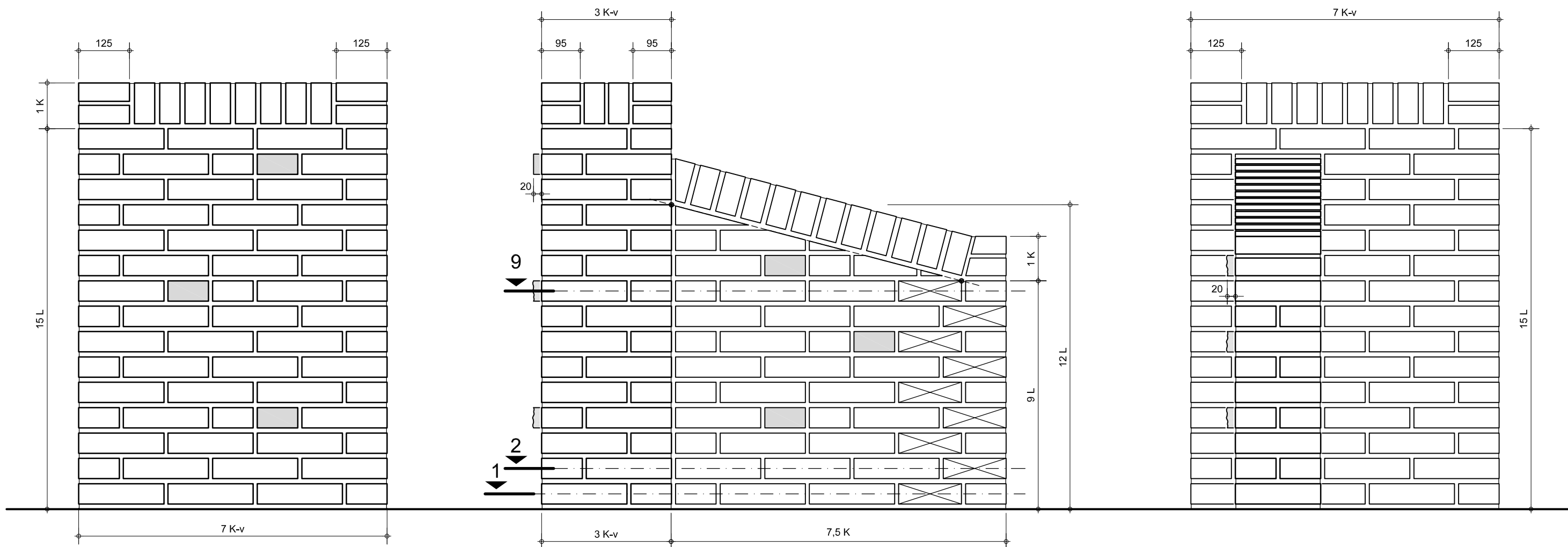
Linker zijaanzicht
