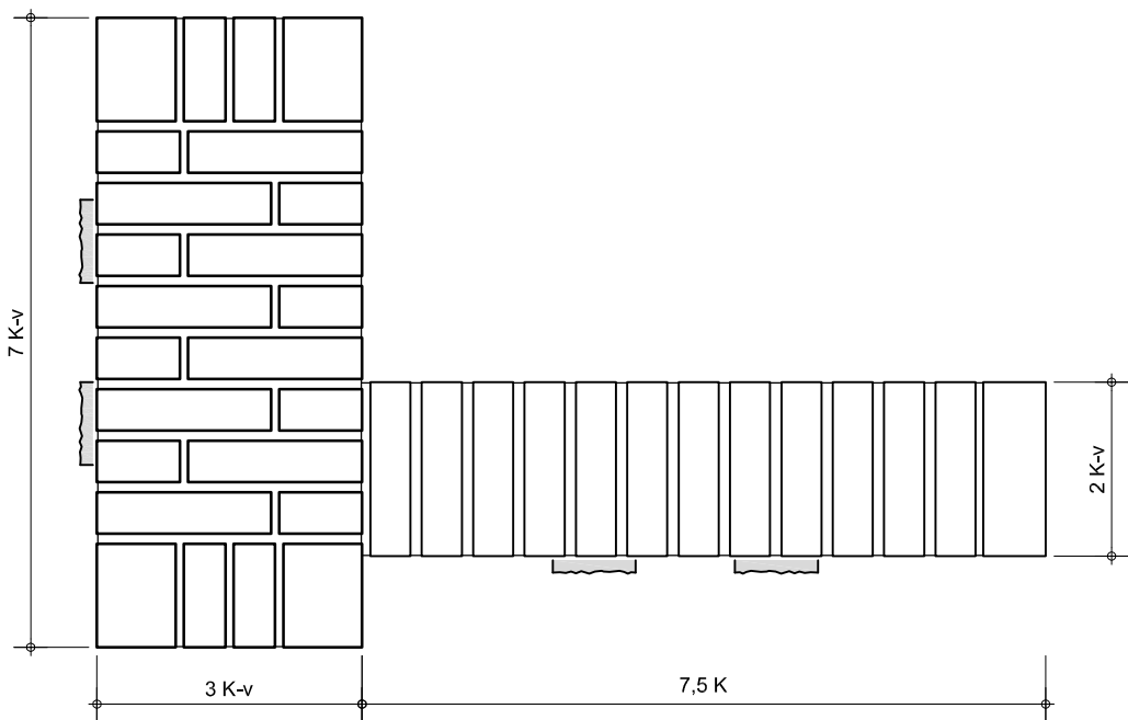
Boven aanzicht
