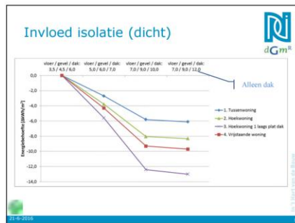
Figuur 1: Invloed isolatie grondgebonden woningen op eis energiebehoefte. Boven R_c=9 zeer weinig invloed meer door gevelisolatie.
