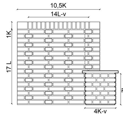
Zijaanzicht Noord
