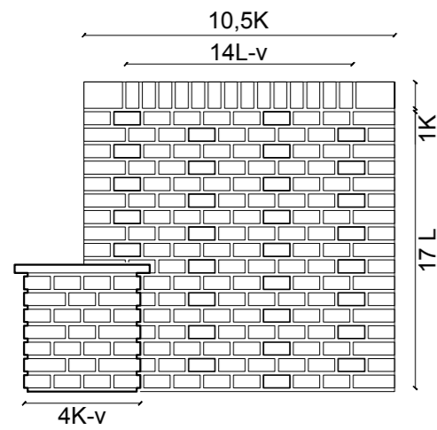
Zijaanzicht Zuid
