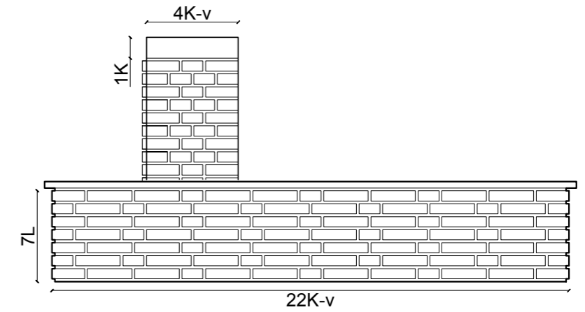
Achteraanzicht
