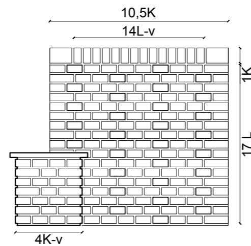
Zijaanzicht Noord
