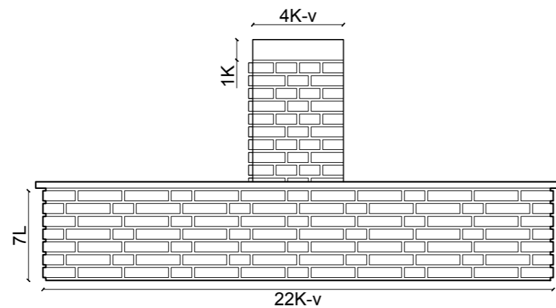
Vooraanzicht
