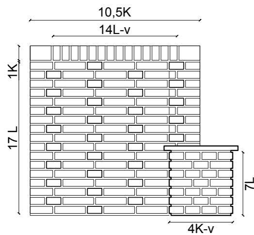
Zijaanzicht Zuid
