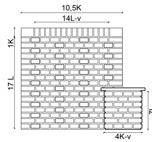
Zijaanzicht Noord
