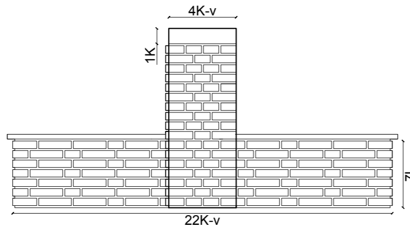
Vooraanzicht
