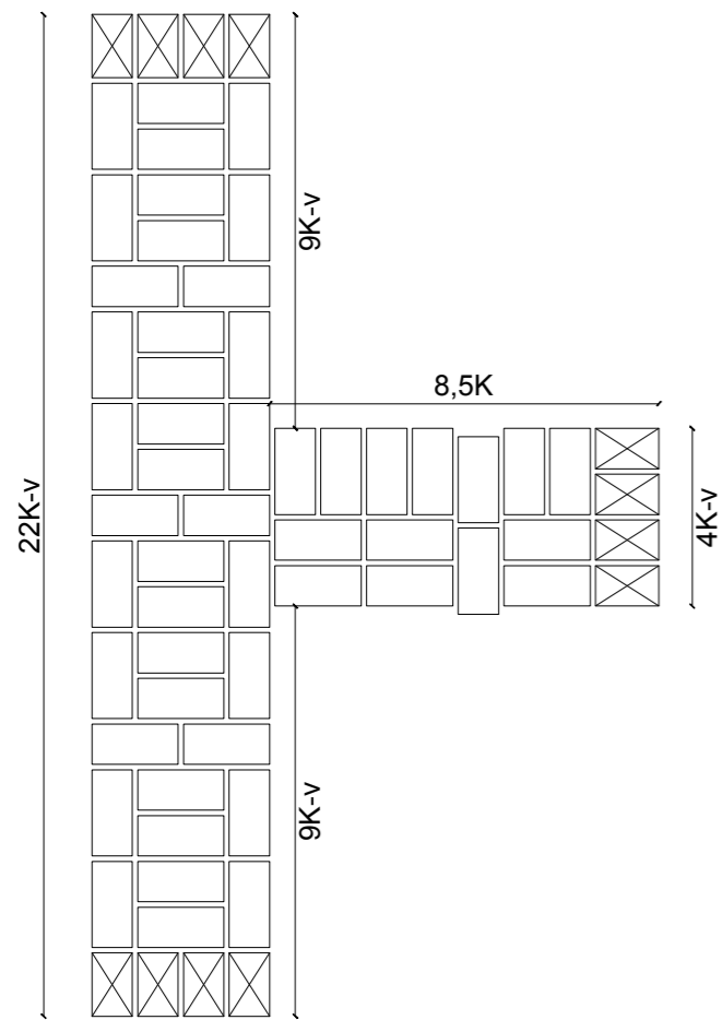
Lagen 1, 3, 5, 7
