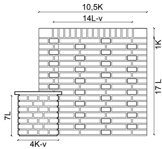
Zijaanzicht Zuid
