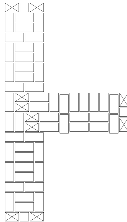
Lagen 2, 4, 6
