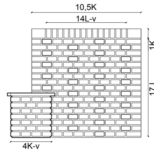
Zijaanzicht Noord
