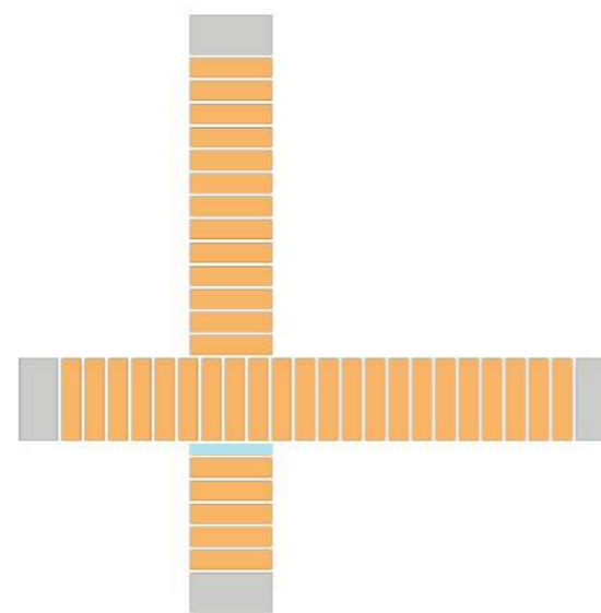
laag 12 (rollaag)
