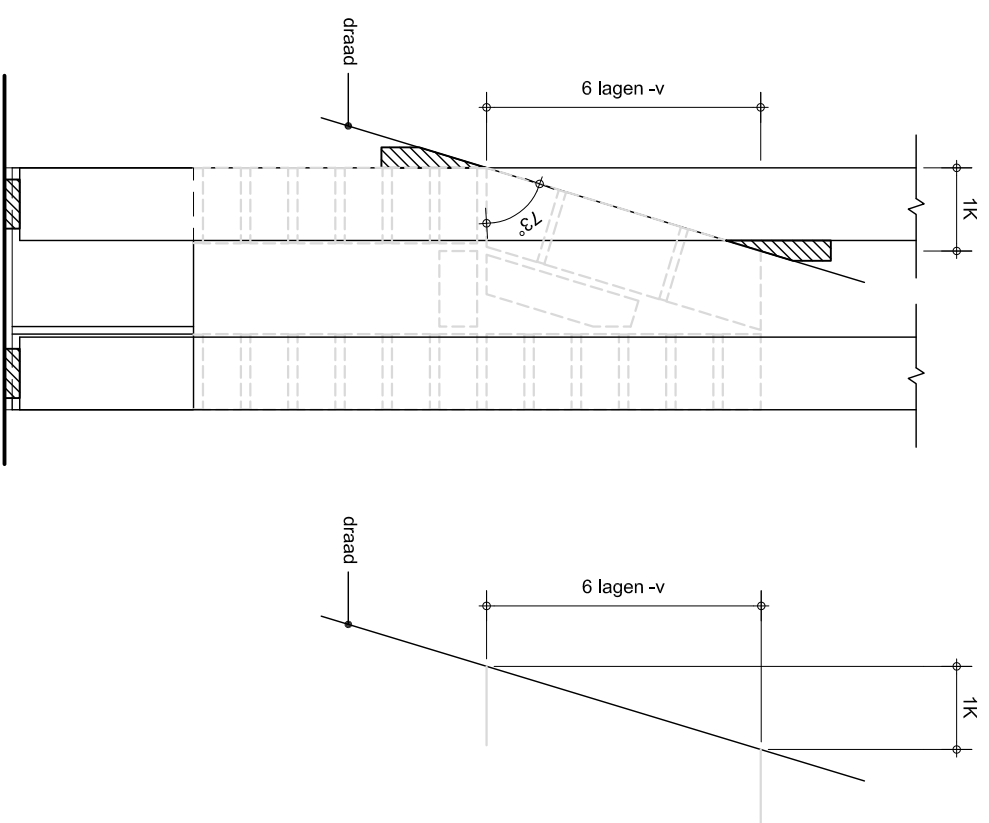
Rechter zijaanzicht
