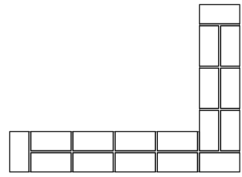
Laag 1 en 9
