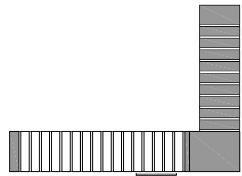
Bovenaanzicht
